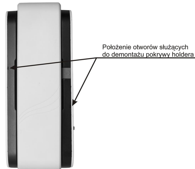
Rys 2. Rozmieszczenie otworów w pokrywie holdera aparatu – służących do demontażu obudowy.
