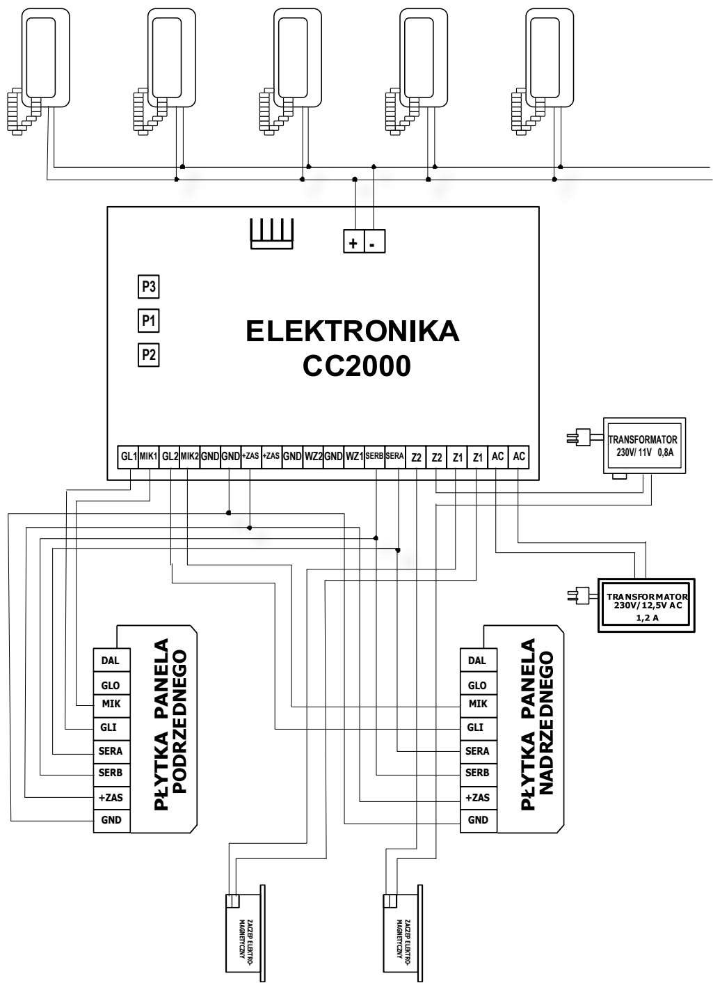
Rys. 6. Schemat ideowy połączeń panelu nadrzędnego i podrzędnego w systemie CC-2000.
