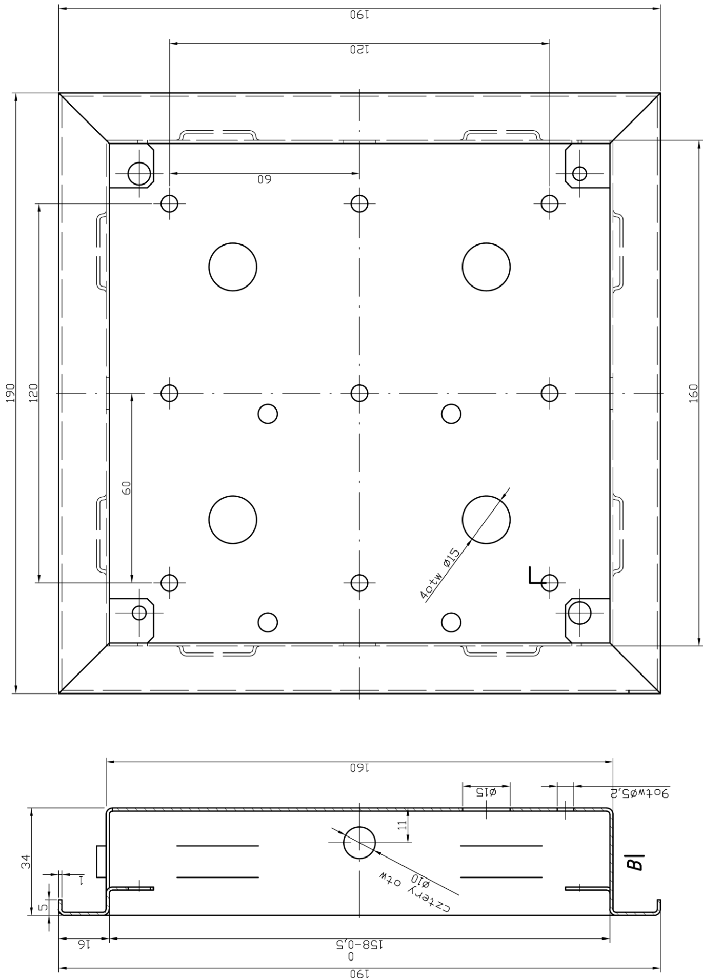
Rys. 3a. Wymiary ramki podtynkowej panelu PC-2000
