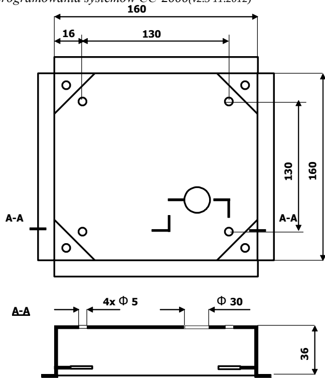
Rys. 3b. Wymiary ramki podtynkowej panelu PC-1000
