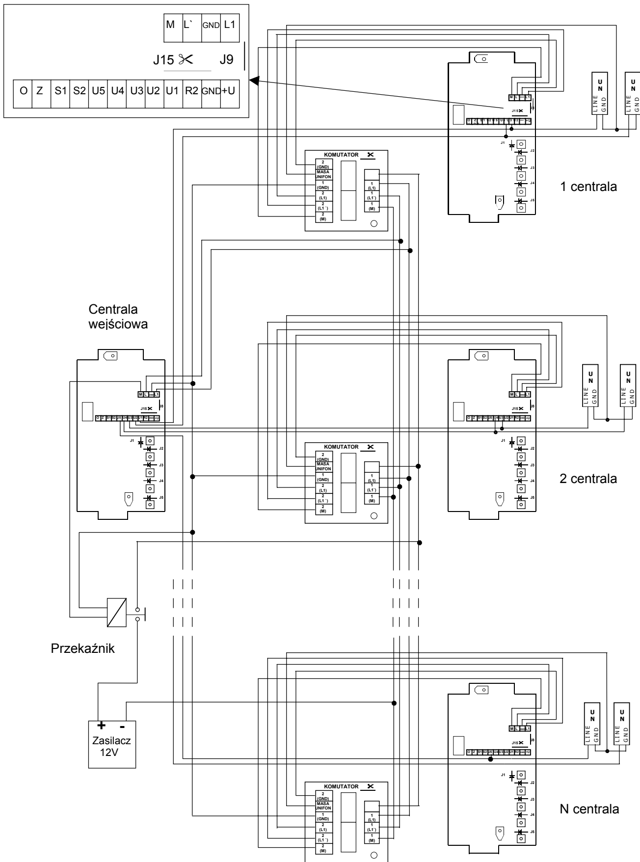
Schemat podłączenia komutatorów do central TD-6 pracujących w konfiguracji: 1 centrala zewnętrzna - N central wewnętrznych
