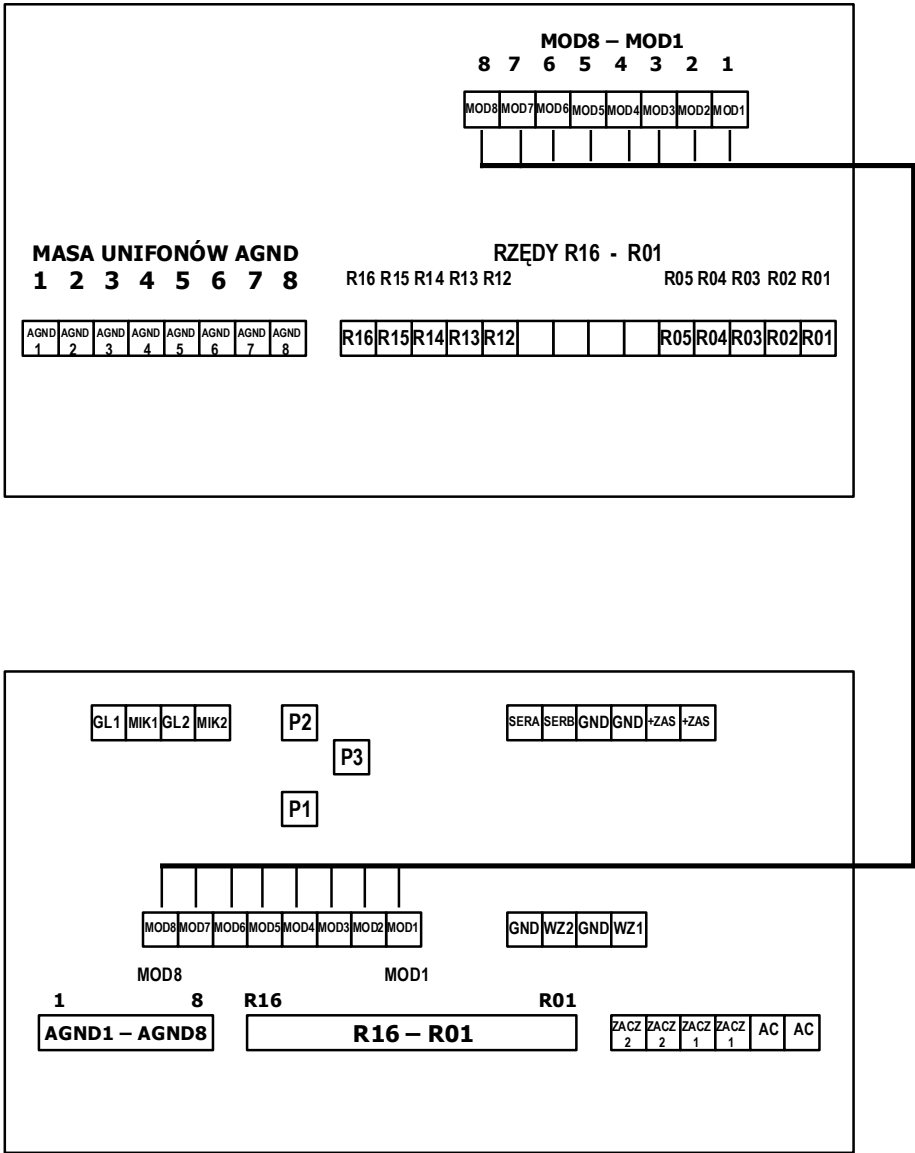
Rys. 11. Schemat podłączenia rozszerzenia na przykładzie elektroniki systemu CC-1000
