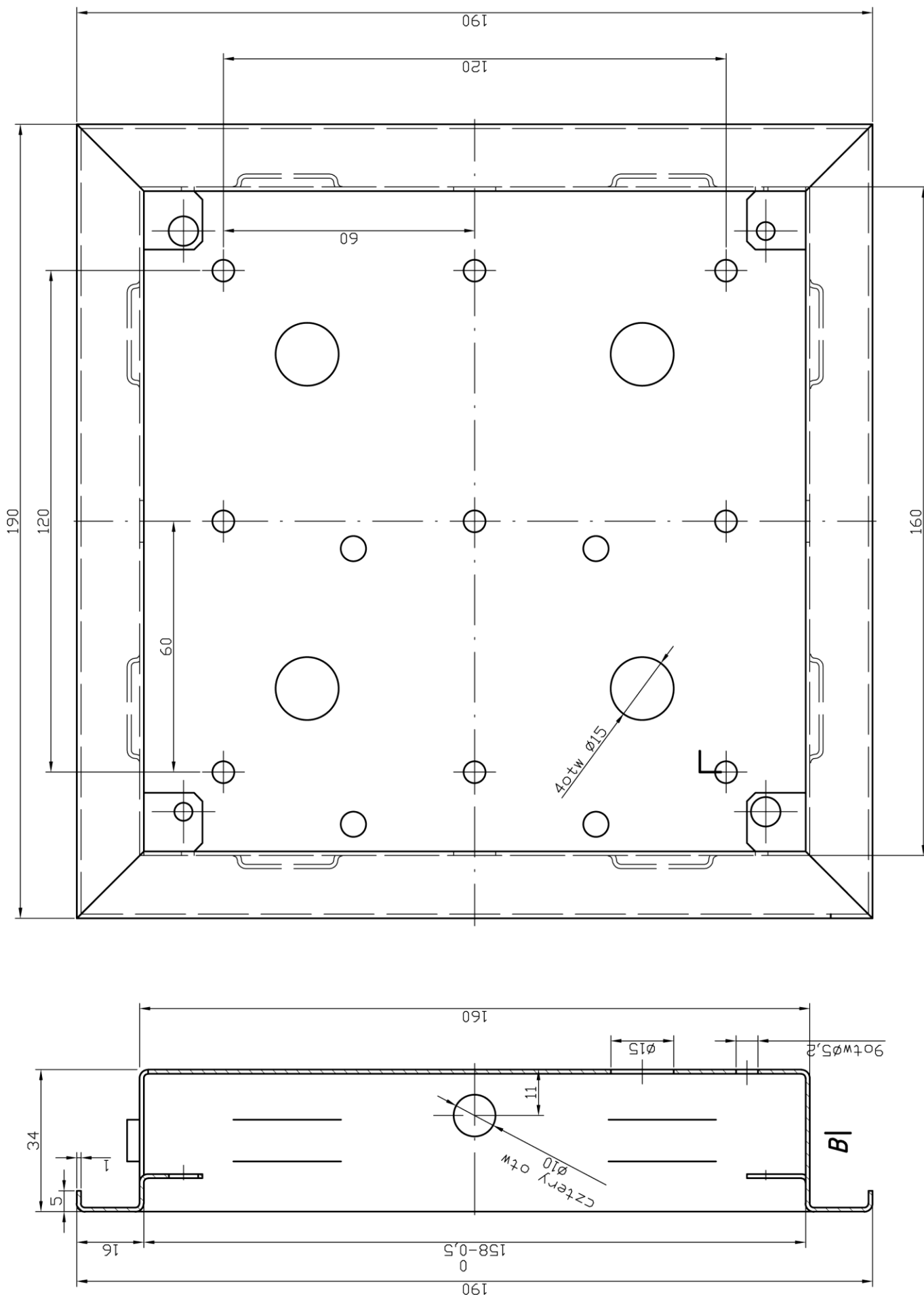
Rys. 1b. Wymiary ramki podtynkowej panela PC-2000
