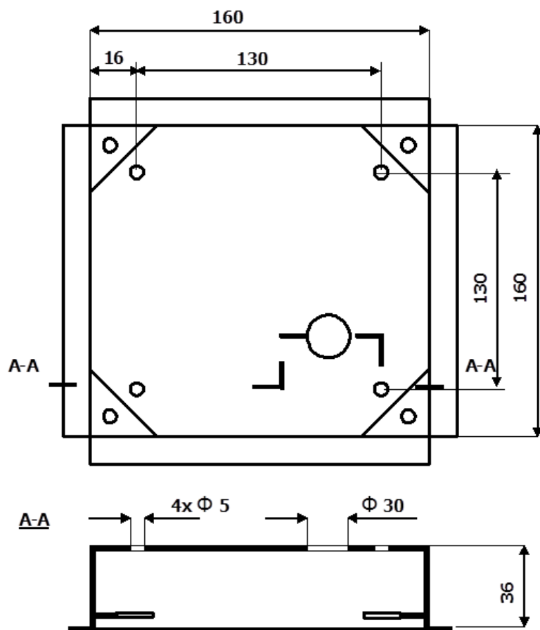
Rys. 1a. Wymiary ramki podtynkowej panela PC-1000
