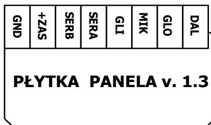
Rys. 3. Widok złącza panela PC-1000 i PC-2000
