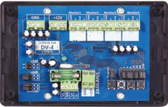
Dystrybutor DV-4 w plastikowej obudowie
