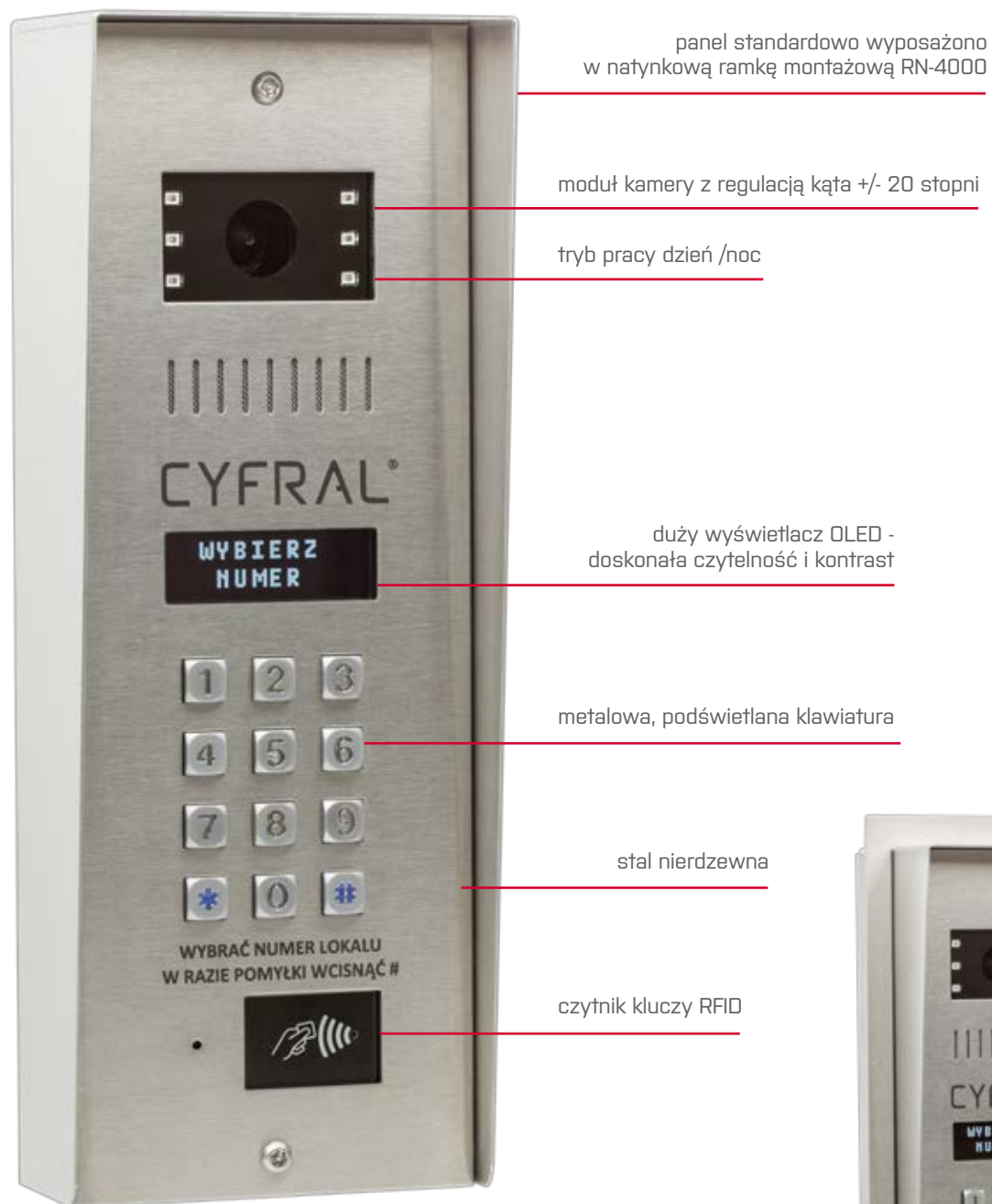
■ Panel rozmówny PC-4000RV, montaż natynkowy
